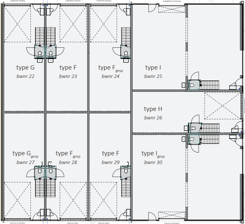
begane grond
