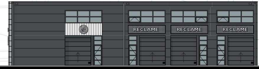
noordgevel
