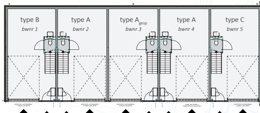
begane grond
