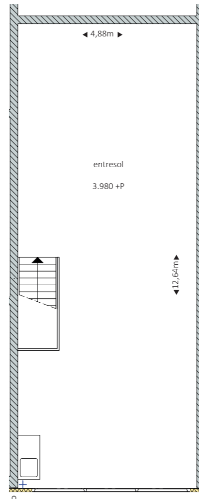
verdieping
