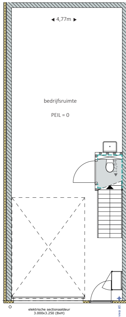
begane grond
