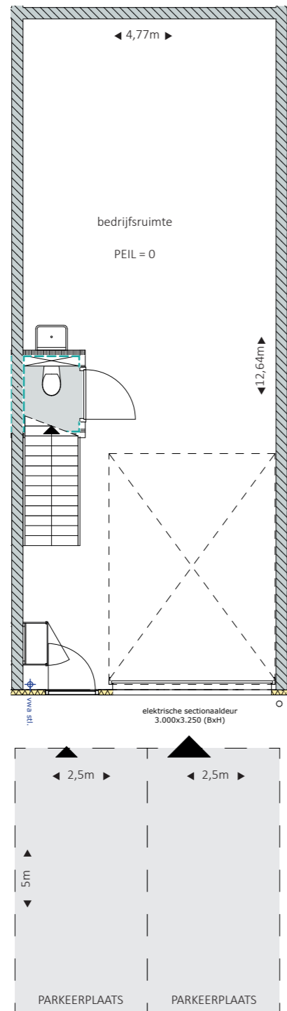
begane grond
